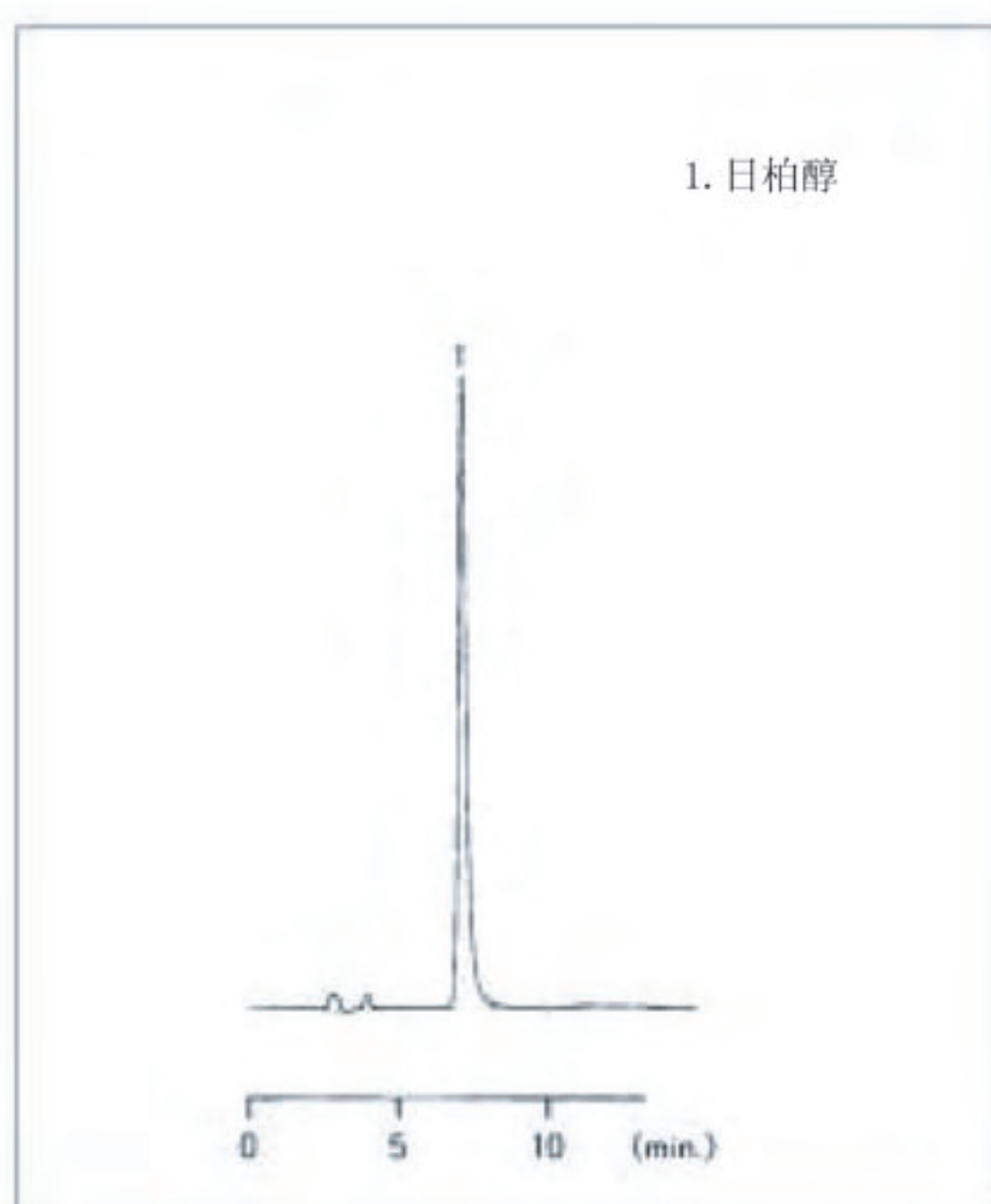
日柏醇标准品的色谱图
